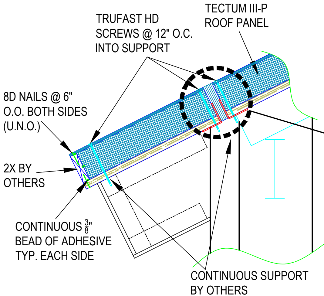
1 TECTUM III-P - OVER EXTERIOR WALL Scale: N.T.S.
