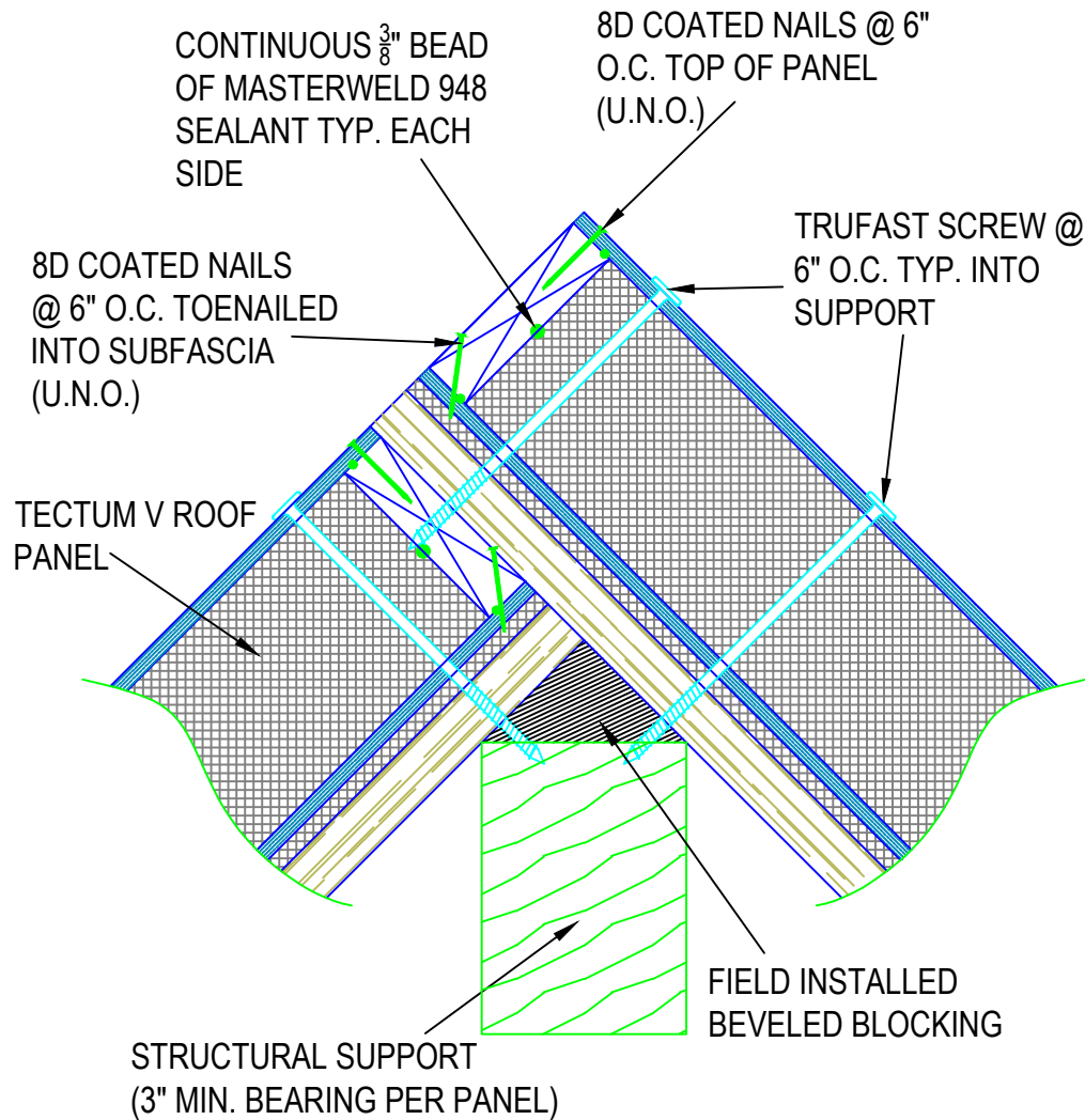
1 TECTUM V - 12:12 RIDGE DETAIL Scale: N.T.S.
