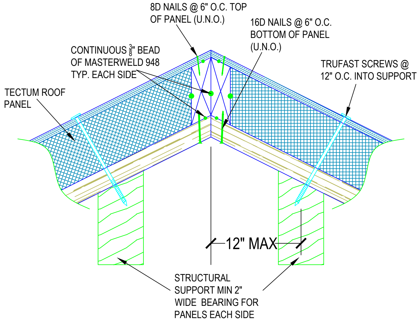
1 CANTILEVERED RIDGE Scale: N.T.S.
