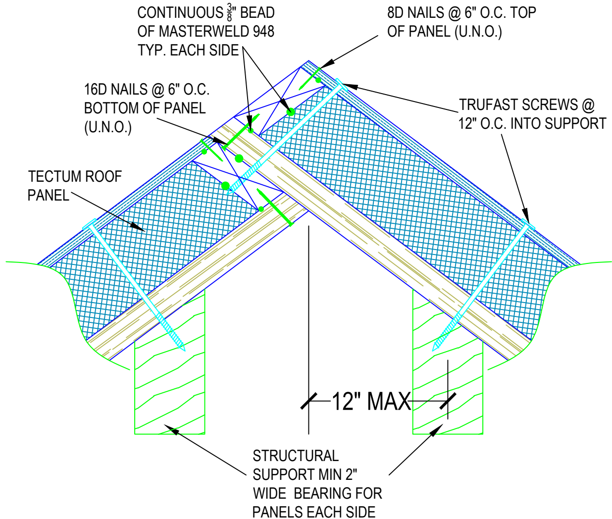
1 OVERLAY CANTILEVERED RIDGE Scale: N.T.S.
