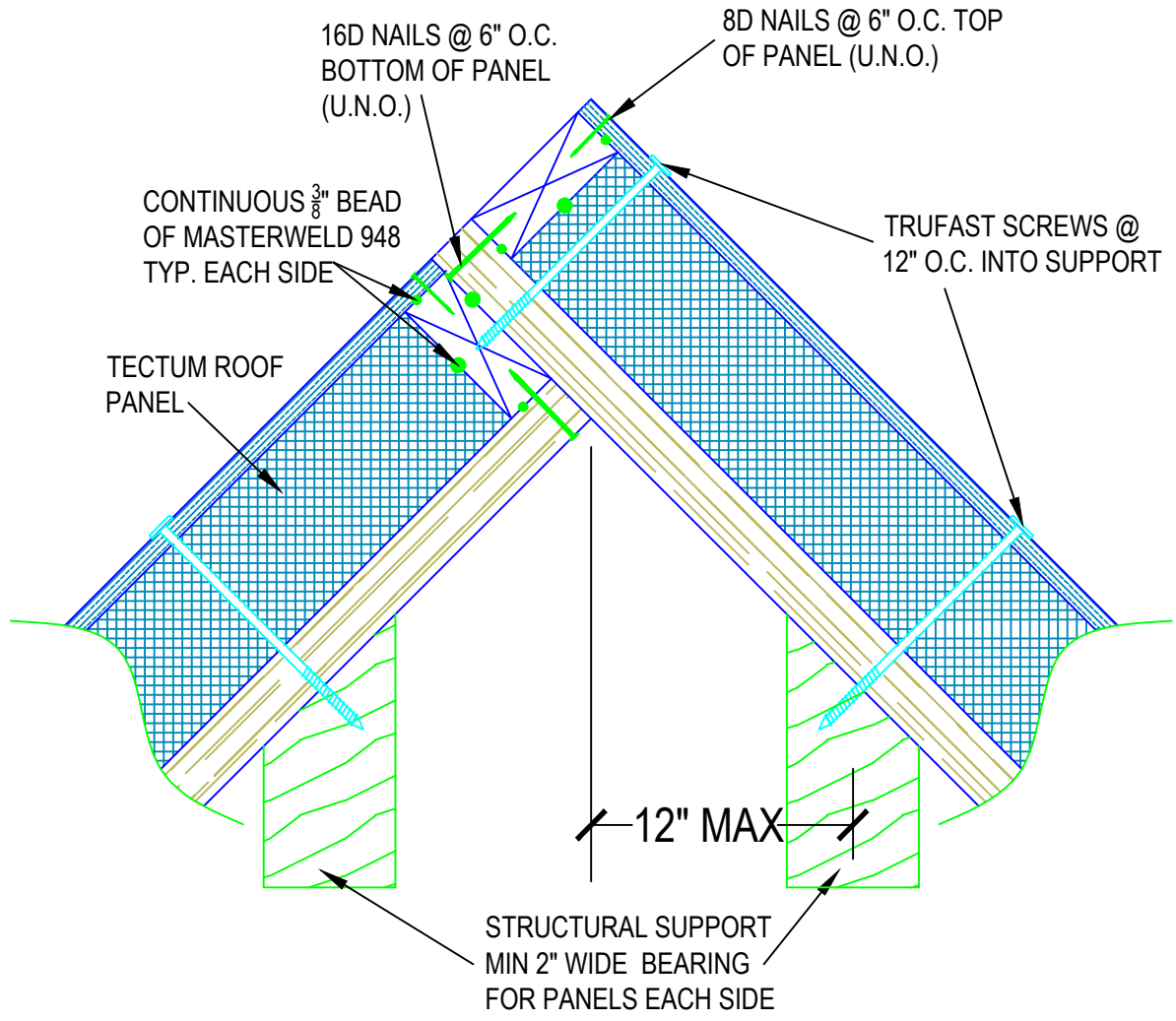
1 12:12 CANTILEVERED RIDGE DETAIL Scale: N.T.S.
