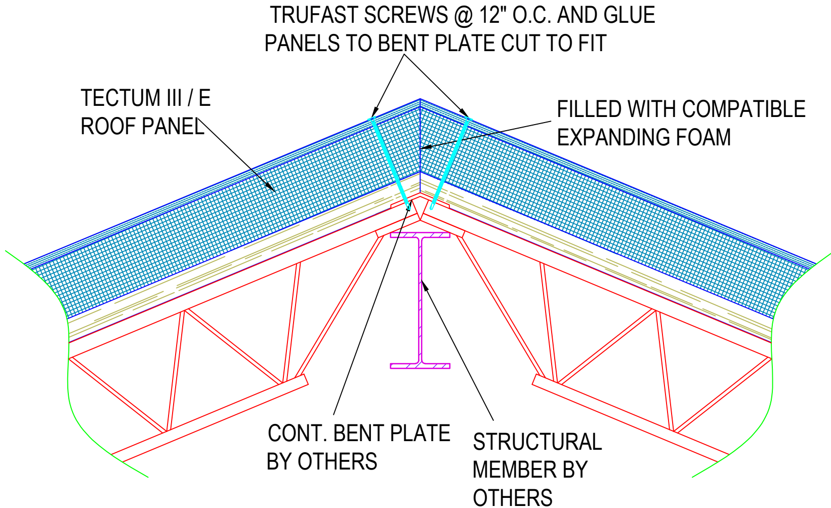
1 RIDGE ON STEEL JOIST Scale: N.T.S.
