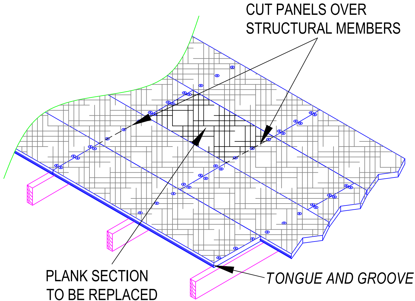
1 REMOVING TECTUM ROOF PLANK Scale: N.T.S.
