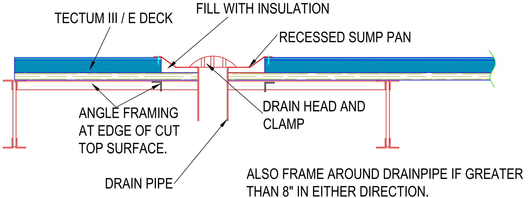
1 SUMP DETAIL III & E Scale: N.T.S.
