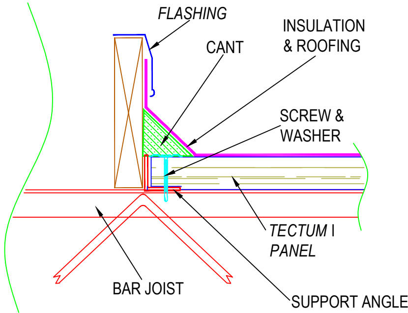
1 TECTUM I FLUSH TO PARAPET Scale: N.T.S.
